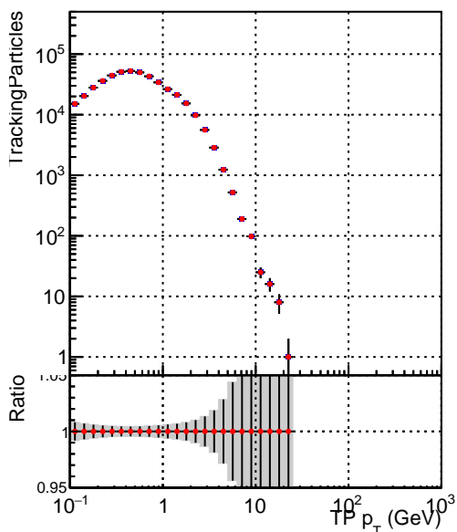
■ SoftQCD_default ● SoftQCD_ckfPixelLessStep
