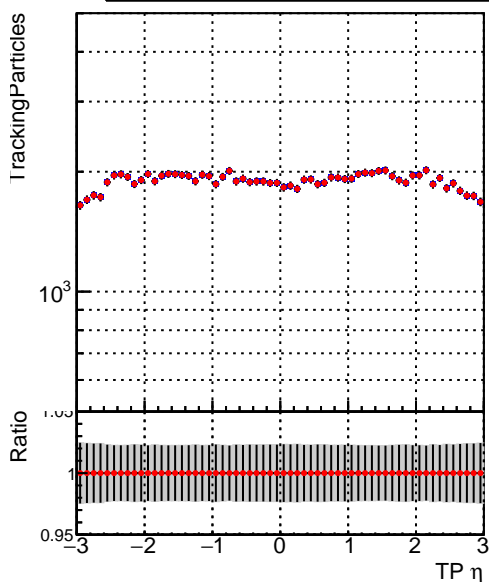
■ SoftQCD_default ● SoftQCD_ckfPixelLessStep
