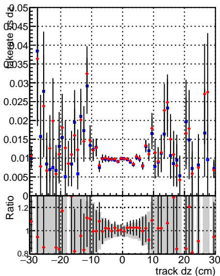
Fake rate vs dz —●— SoftQCD_default —●— SoftQCD_ckfPixelLessStep
