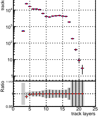
SoftQCD_ckfPixelLessStep
