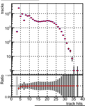
SoftQCD_default
