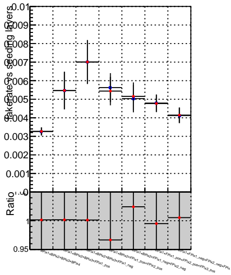
—● SoftQCD_default —● SoftQCD_ckfPixelLessStep
