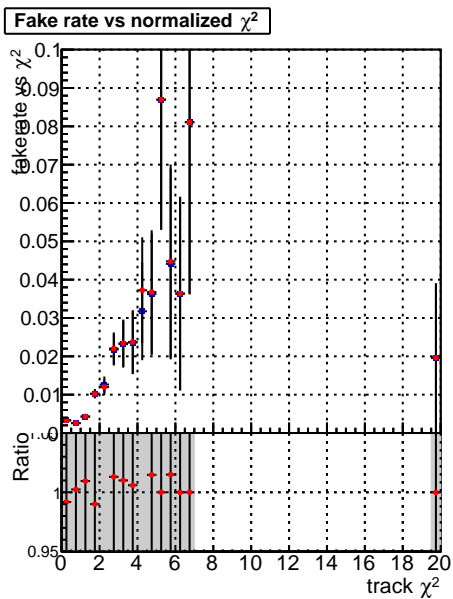
—● SoftQCD_default —● SoftQCD_ckfPixelLessStep
