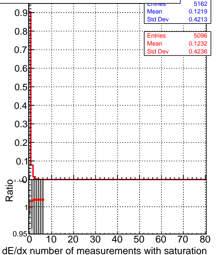
■ SoftQCD_default ◆ SoftQCD_ckfPixelLessStep
