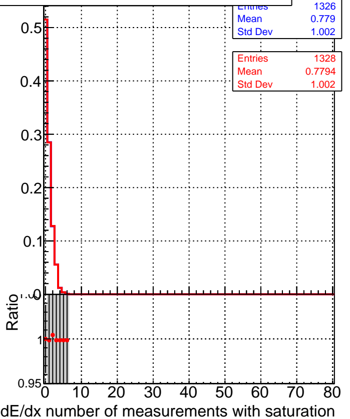
■ SoftQCD_default ● SoftQCD_ckfPixelLessStep
