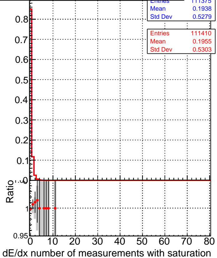
■ SoftQCD_default ● SoftQCD_ckfPixelLessStep
