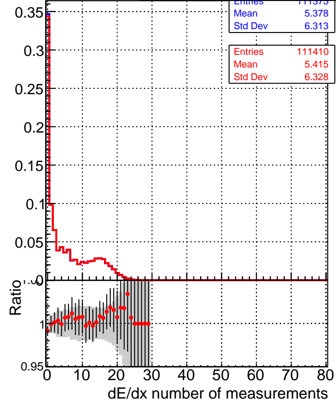
■ SoftQCD_default ● SoftQCD_ckfPixelLessStep
