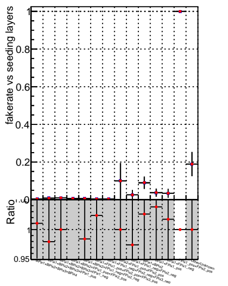
—◆— SoftQCD_default —●— SoftQCD_ckfPixelLessStep
