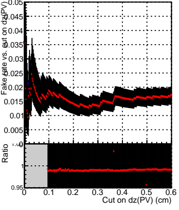
—● SoftQCD_default —● SoftQCD_ckfPixelLessStep
