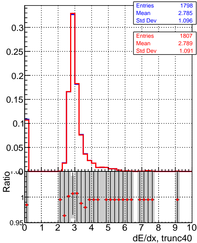
■ SoftQCD_default ● SoftQCD_ckfPixelLessStep
