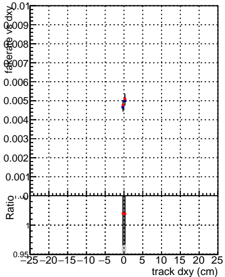
SoftQCD_default SoftQCD_ckfPixelLessStep
