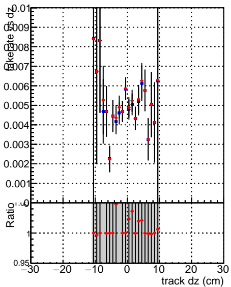
SoftQCD_default SoftQCD_ckfPixelLessStep
