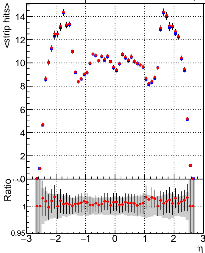
SoftQCD_default SoftQCD_ckfPixelLessStep
