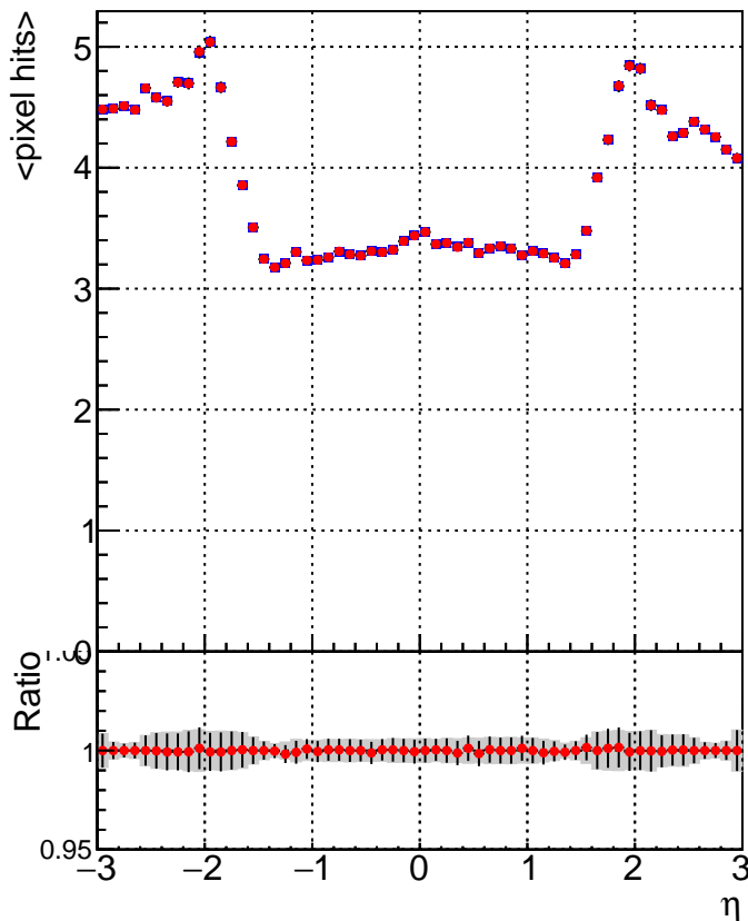
SoftQCD_default SoftQCD_ckfPixelLessStep
