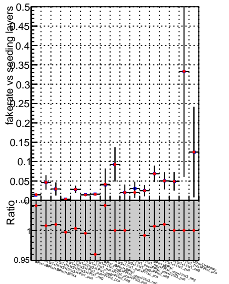
Fake rate vs. ◆ SoftQCD_default ● SoftQCD_ckfPixelLessStep
