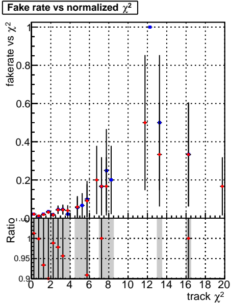
Fake rate vs. ◆ SoftQCD_default ● SoftQCD_ckfPixelLessStep
