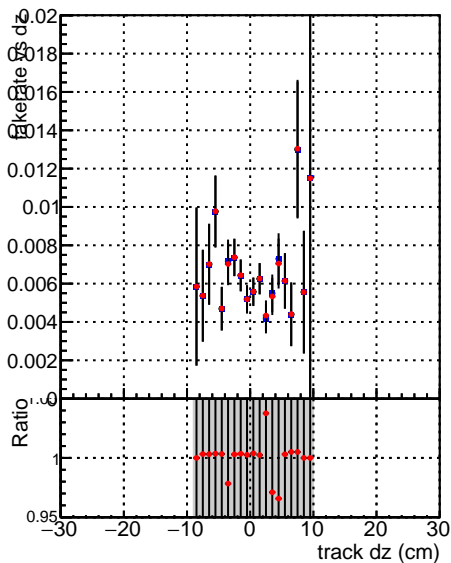
—●— SoftQCD_default —●— SoftQCD_ckfPixelLessStep
