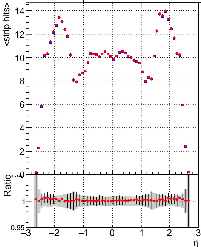
SoftQCD_default SoftQCD_ckfPixelLessStep
