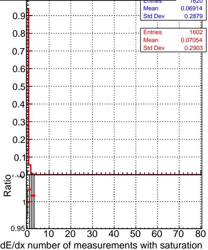
■ SoftQCD_default ◆ SoftQCD_ckfPixelLessStep
