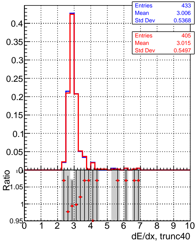
■ SoftQCD_default ● SoftQCD_ckfPixelLessStep
