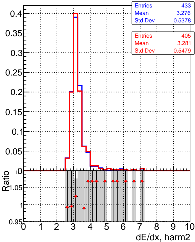
■ SoftQCD_default ● SoftQCD_ckfPixelLessStep
