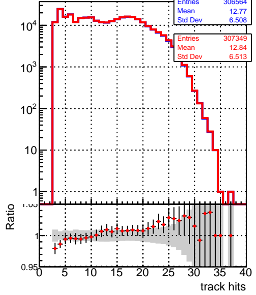
track hits — SoftQCD_default — SoftQCD_ckfPixelLessStep
