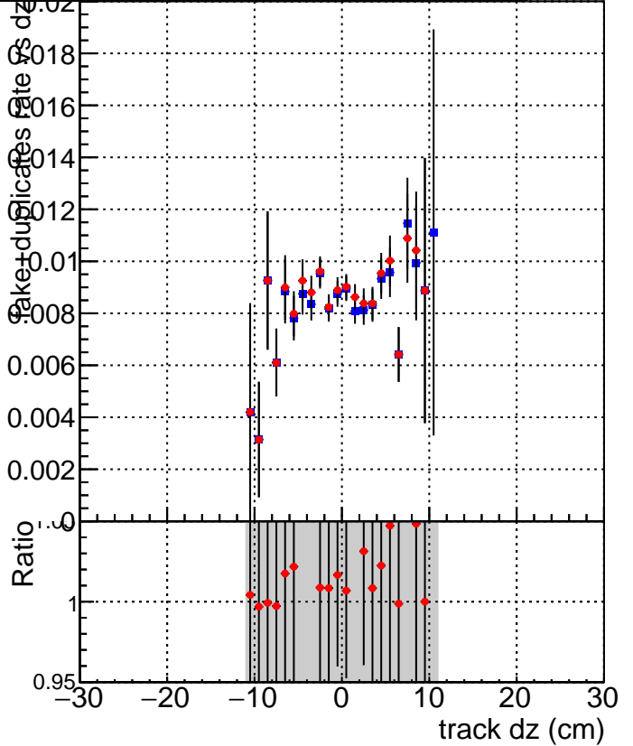
SoftQCD_default SoftQCD_ckfPixelLessStep
