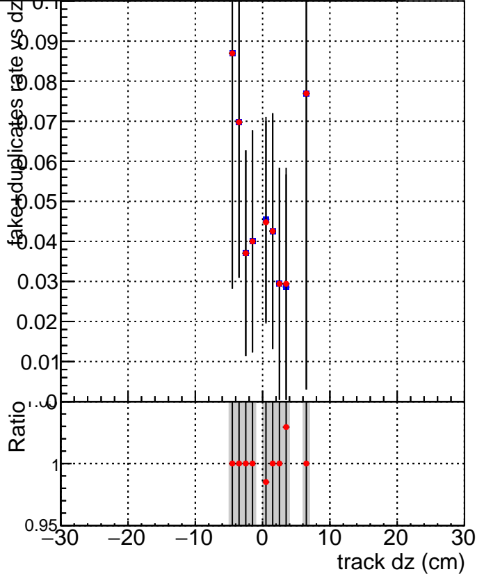
SoftQCD_default SoftQCD_ckfPixelLessStep
