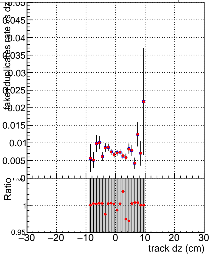
SoftQCD_default SoftQCD_ckfPixelLessStep
