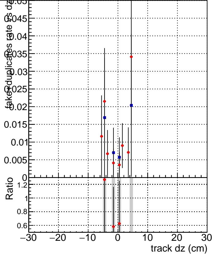
SoftQCD_default SoftQCD_ckfPixelLessStep
