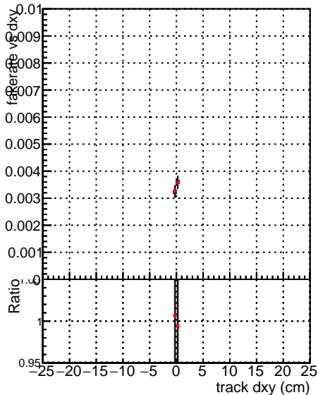
—●— SoftQCD_default —●— SoftQCD_ckptPixelLessStep
