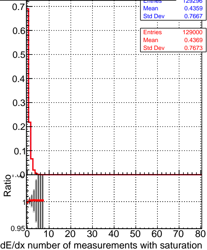
■ SoftQCD_default ◆ SoftQCD_ckfPixelLessStep
