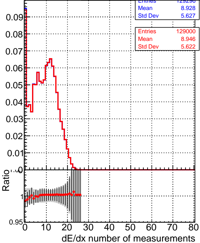
■ SoftQCD_default ◆ SoftQCD_ckfPixelLessStep
