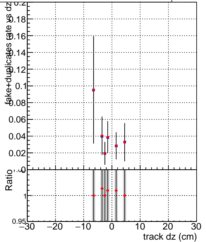
SoftQCD_default SoftQCD_ckfPixelLessStep
