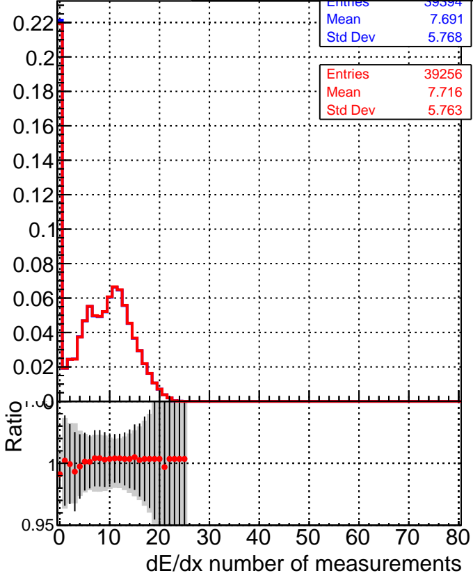
— SoftQCD_default — SoftQCD_ckfPixelLessStep
