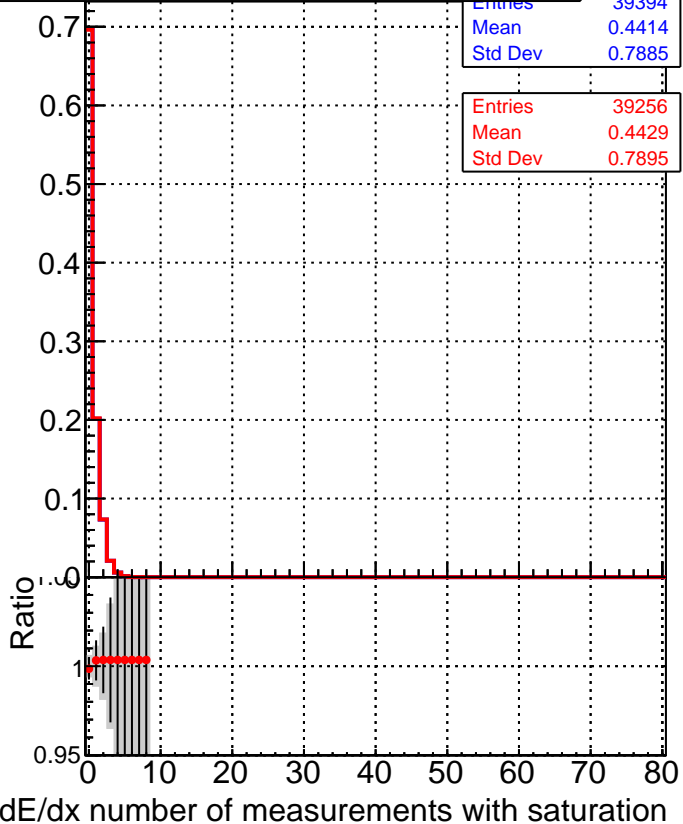
— SoftQCD_default — SoftQCD_ckfPixelLessStep
