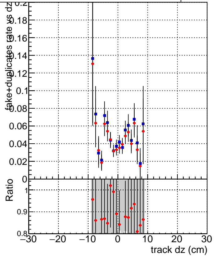
SoftQCD_default SoftQCD_ckfPixelLessStep
