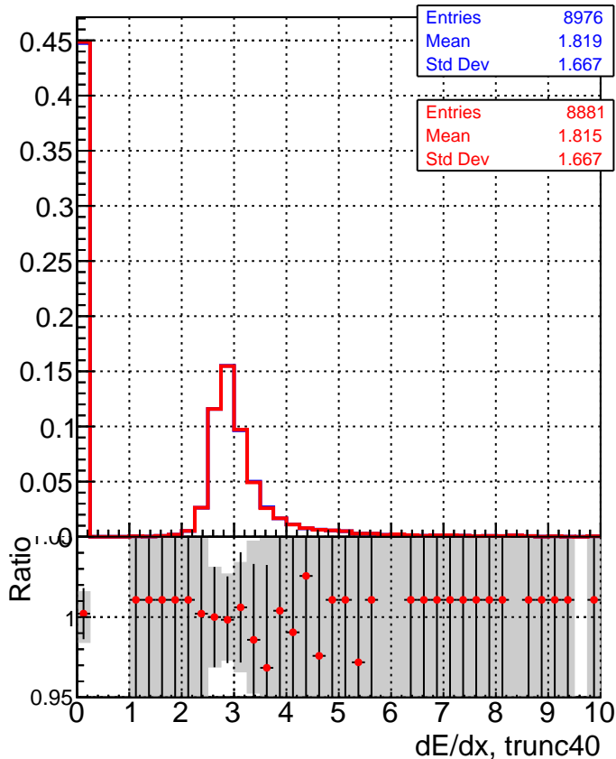
■ SoftQCD_default ● SoftQCD_ckfPixelLessStep
