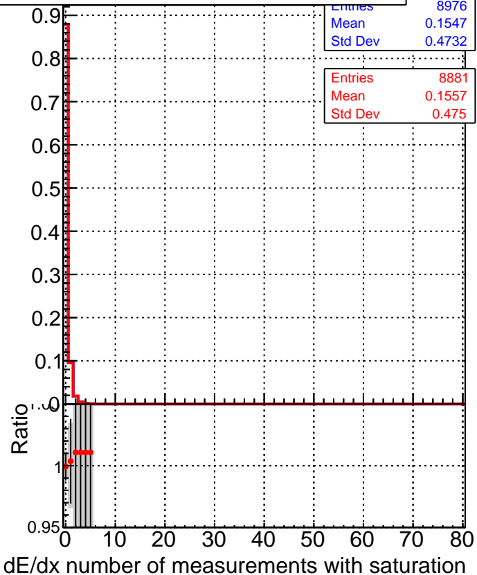
■ SoftQCD_default ● SoftQCD_ckfPixelLessStep
