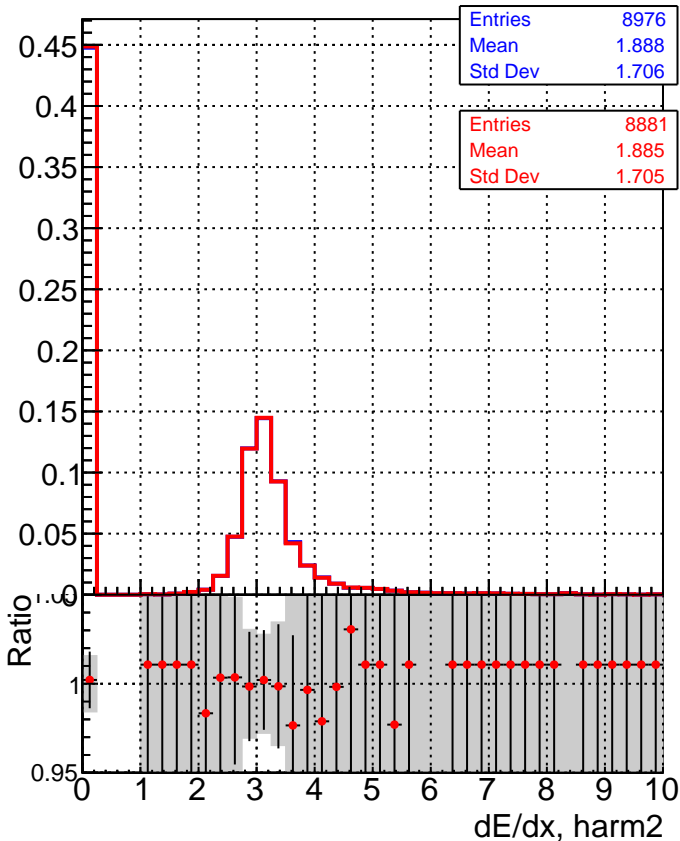
■ SoftQCD_default ● SoftQCD_ckfPixelLessStep
