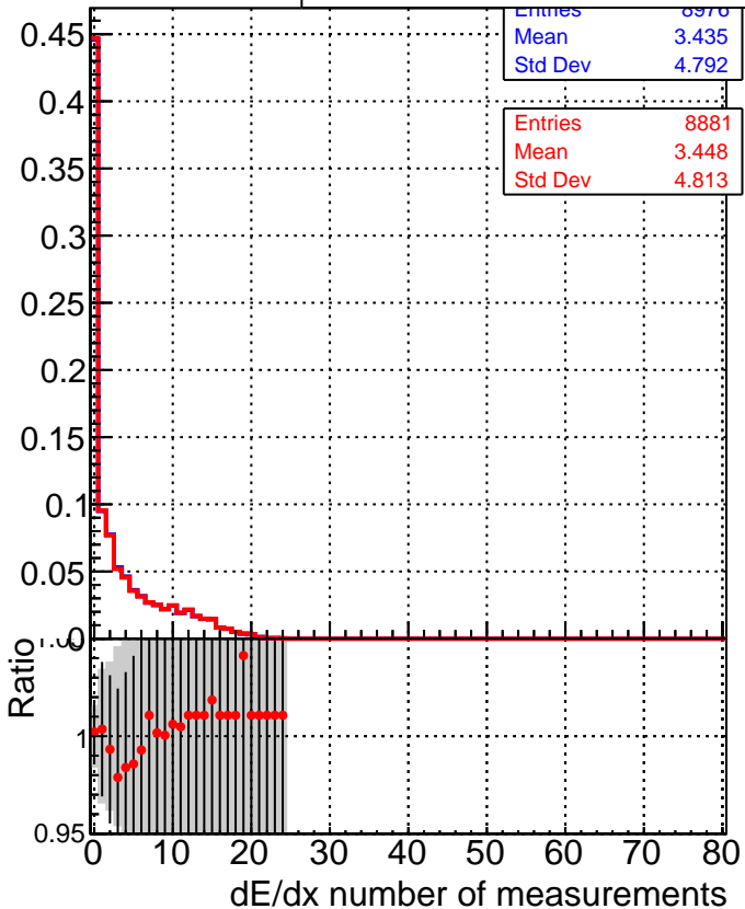
■ SoftQCD_default ● SoftQCD_ckfPixelLessStep
