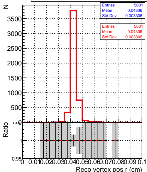
Recons SoftQCD_default
