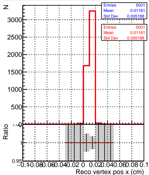
Recons SoftQCD_default
