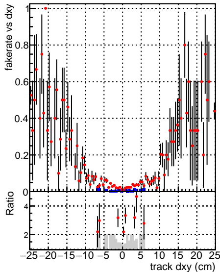
—● SoftQCD_default —● SoftQCD_ckfPixelLessStep
