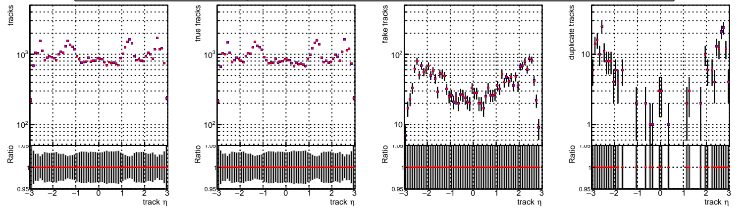
—●— SoftQCD_default —●— SoftQCD_ckfPixelLessStep
