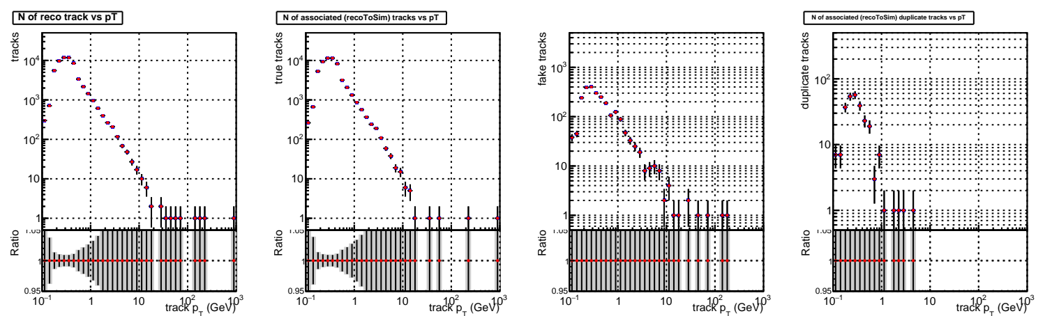
—●— SoftQCD_default —●— SoftQCD_ckfPixelLessStep
