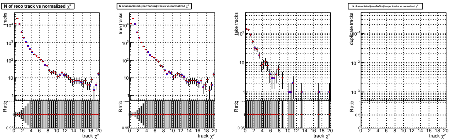
N of reco track vs. \chi^2 —●— SoftQCD_default —●— SoftQCD_ckptPixelLessStep
