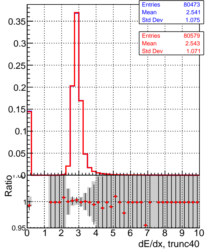
■ SoftQCD_default ● SoftQCD_ckfPixelLessStep
