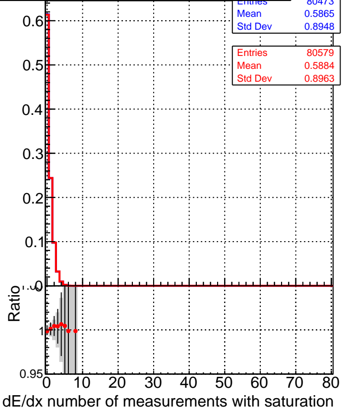
■ SoftQCD_default ● SoftQCD_ckfPixelLessStep
