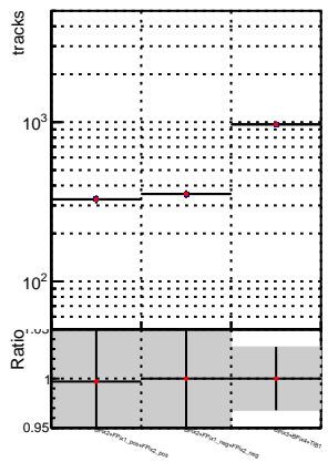
N of reco track vs. \chi^2 —●— SoftQCD_default —●— SoftQCD_ckfPixelLessStep
