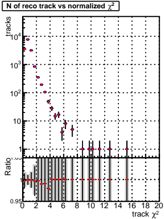
N of reco track vs. \chi^2 SoftQCD_default SoftQCD_ckfPixelLessStep
