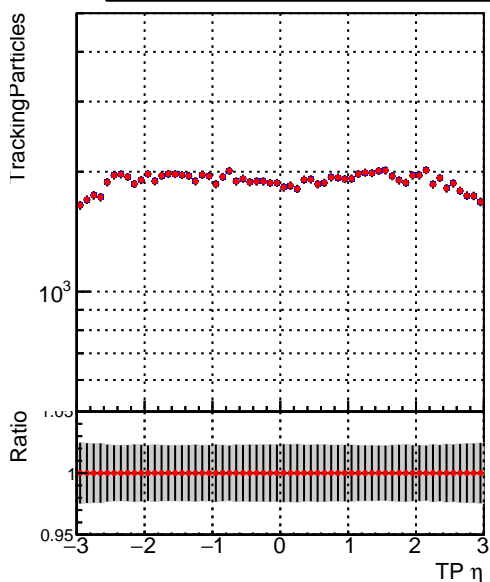
■ SoftQCD_default ■ SoftQCD_ckptPixelLessStep
