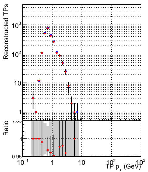
■ SoftQCD_default ■ SoftQCD_ckptPixelLessStep
