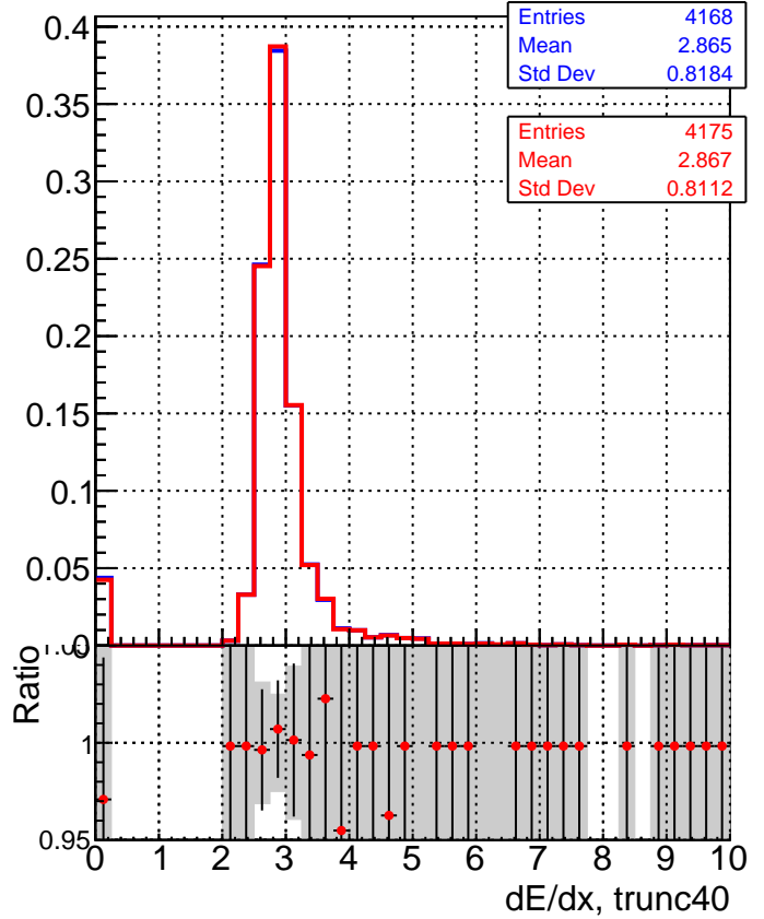
■ SoftQCD_default ● SoftQCD_ckfPixelLessStep
