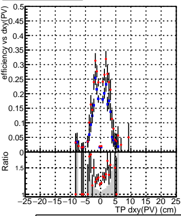
Legend: —●— SoftQCD_default —●— SoftQCD_ckfPixelLessStep
