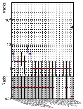
N of reco track vs. \chi^2 —●— SoftQCD_default —●— SoftQCD_ckfPixelLessStep
