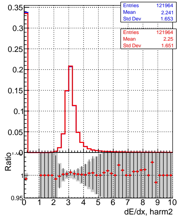
— SoftQCD_default —• SoftQCD_ckfPixelLessStep
