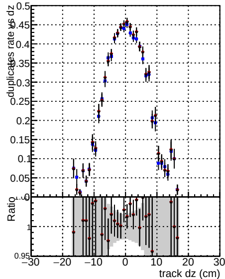
al mkFit100 RECO al mkFit100 tobtec
