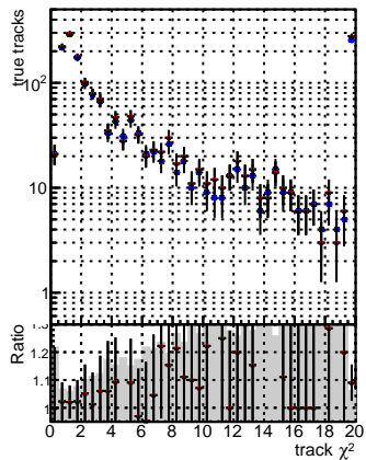
1 Global mkFit100 RECO 1 Global mkFit100 RECO 1 Global mkFit100 RECO
