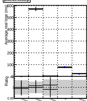
pixelLessStep
