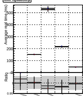
lowPtQuadStep
