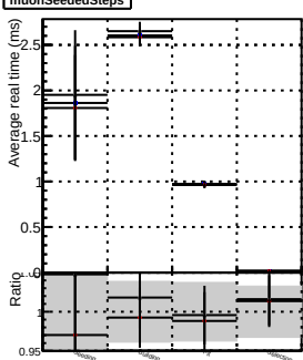
muonSeededSteps
