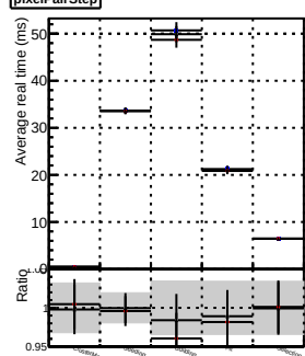
pixelPairStep
