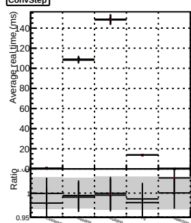
ConvStep
