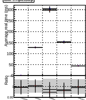
lowPTTripletStep
