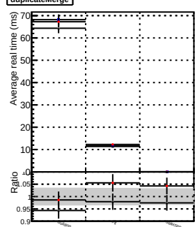
duplicateMerge
