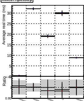
mixedTripletStep
