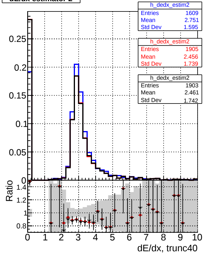
dE/dx estimator 2
