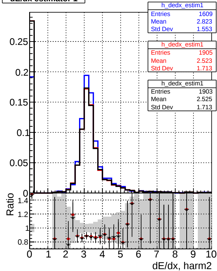
dE/dx estimator 1
