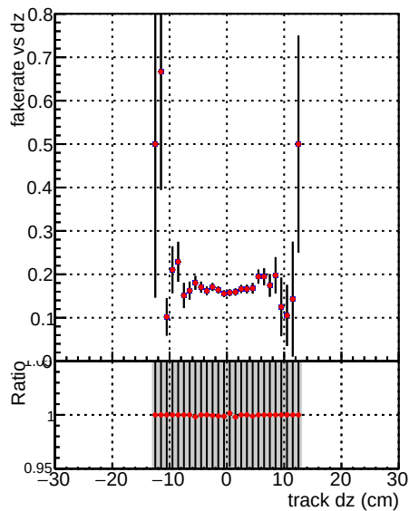
—●— DQM V0001_R000000001 Global mkFit100o RECO —●— DQM V0001_R000000001 Global mkFit100 RECO
