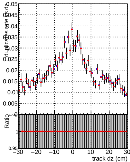
Global mkFit100o RECO
