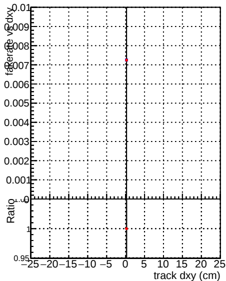
█ DQM_V0001_R0000000001 Global mkFit100o RECO █ DQM_V0001_R0000000001 Global mkFit100dt RECO
