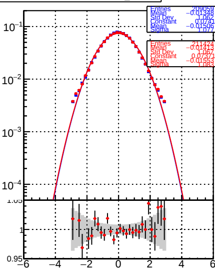
RecoAllAssoc2GenMatched_PulIZ
