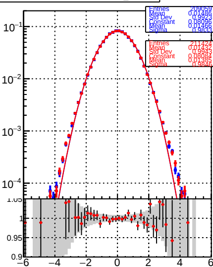
RecoAllAssoc2GenMatched_PulIX
