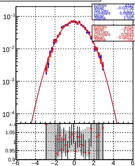
RecoPVAssoc2GenPVMatched_PulIZ
