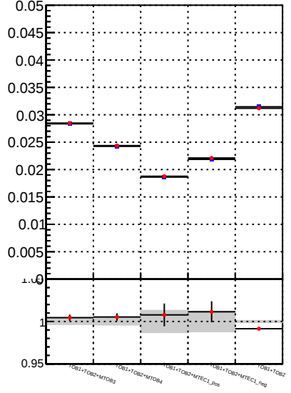
Fake rate vs. —●— DQM TT_mkFit —●— DQM TT_mkFit_BDT
